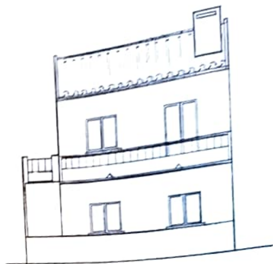
alcado posterior (ampliado)
